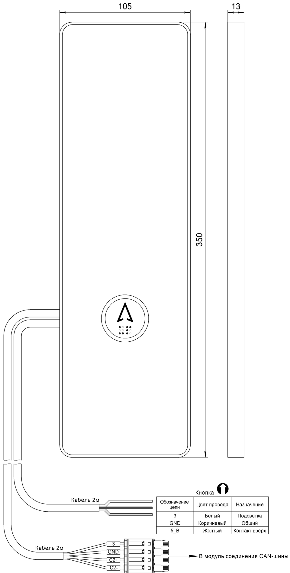
Рис.1 Внешний вид, габаритные и установочные размеры Вызывного поста МАЛАХИТ НШЕК.468381.015
